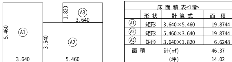
1階 床面積求積図 S:1/200
