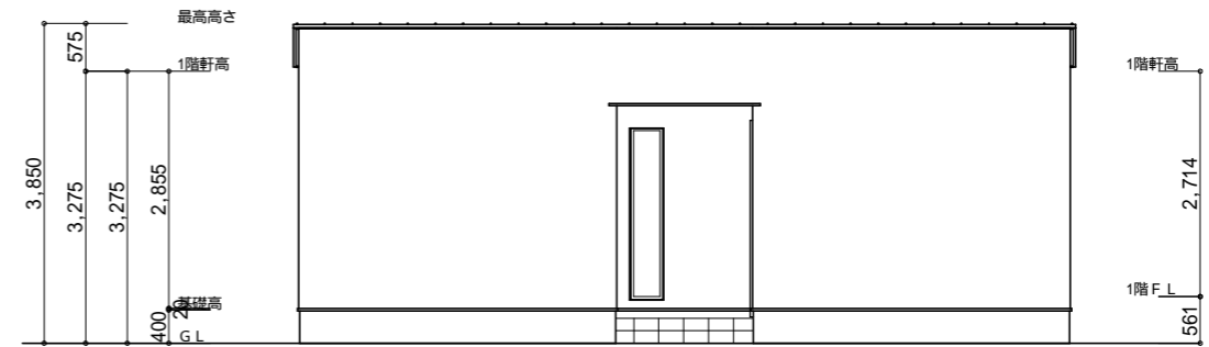
東側 立面図 S:1/100
