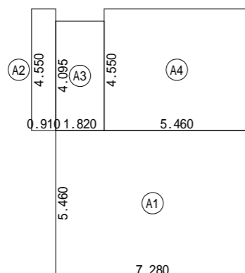
1階 床面積求積図 S:1/200
