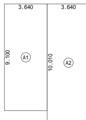
2階 床面積求積図 S:1/200
