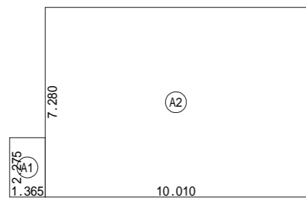
1階 床面積求積図 S:1/200
