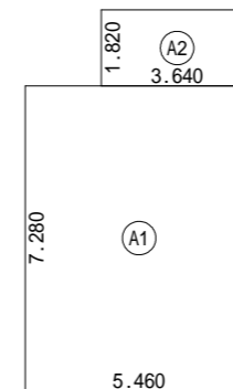
2階 床面積求積図 S:1/200
