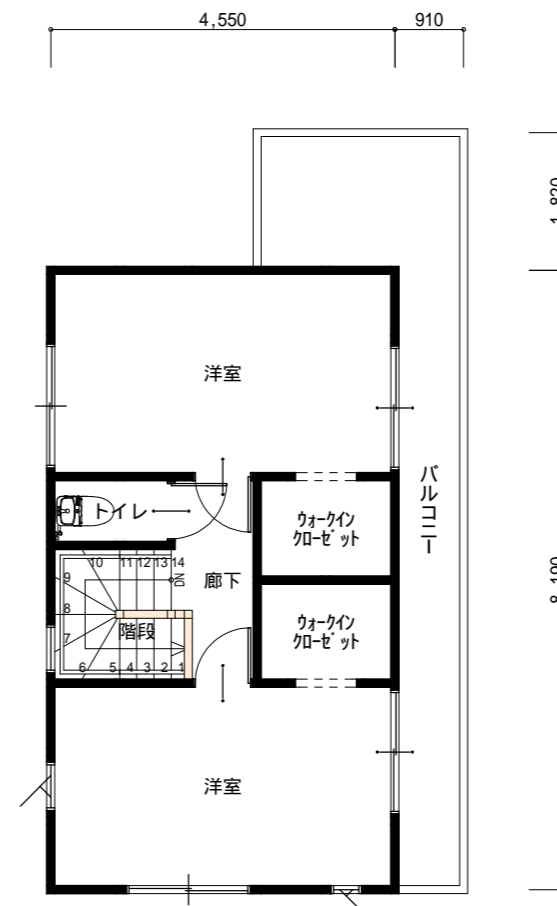
2階 平面図 S:1/100
