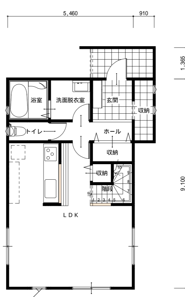
1階 平面図 S:1/100
