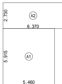
1階 床面積求積図 S:1/200
