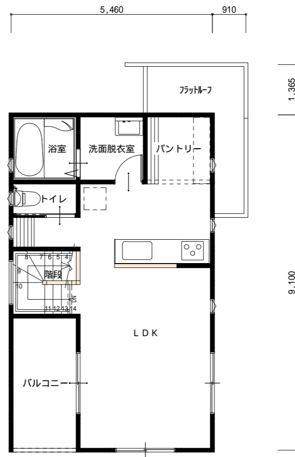
2階 平面図 S:1/100
