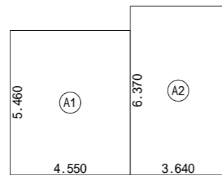
1階 床面積求積図 S:1/200
