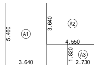
2階 床面積求積図 S:1/200
