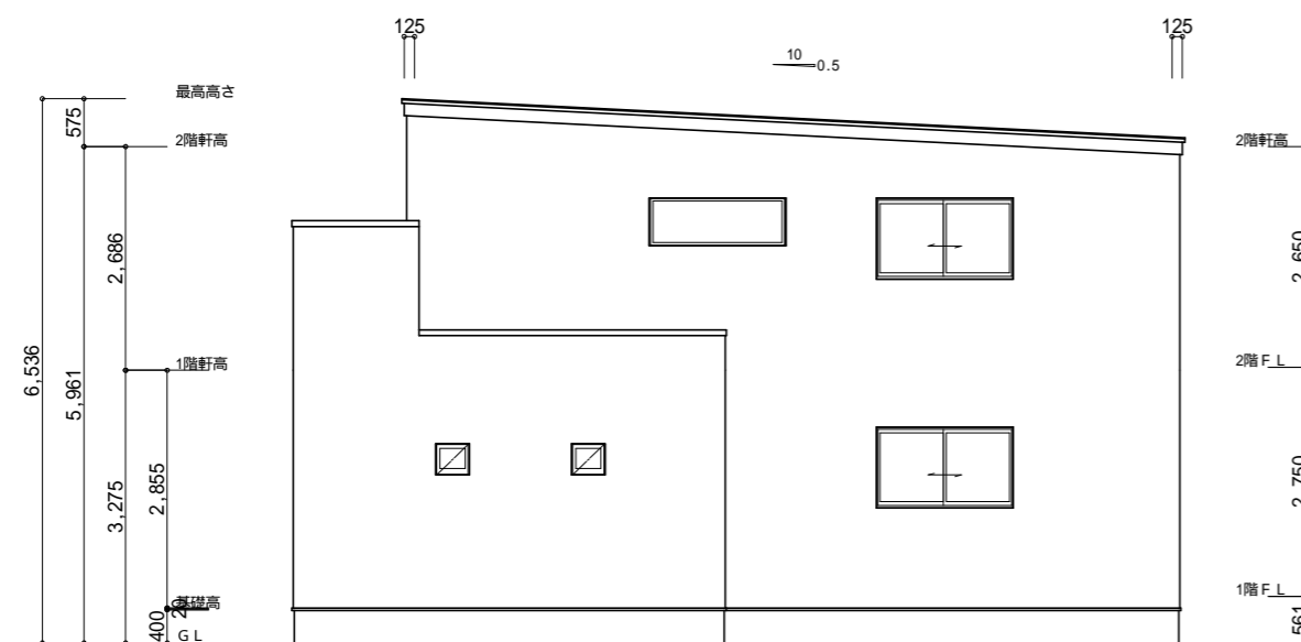
北側 立面図 S:1/100
