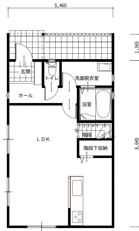
1階 平面図 S:1/100
