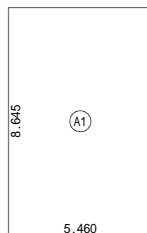
1階 床面積求積図 S:1/200
