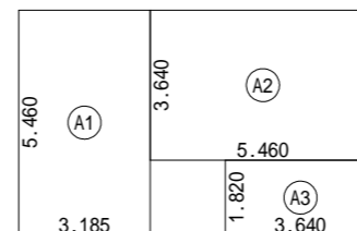
2階 床面積求積図 S:1/200
