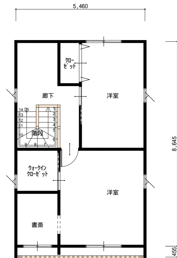
2階 平面図 S:1/100
