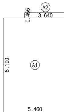
1階 床面積求積図 S:1/200
