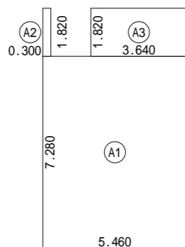
1階 床面積求積図 S:1/200
