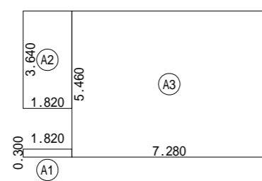
1階 床面積求積図 S:1/200
