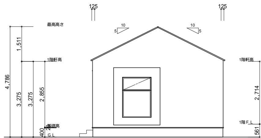
北側 立面図 S:1/100
