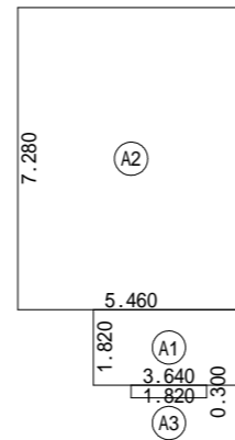
1階 床面積求積図 S:1/200
