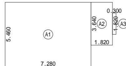
1階 床面積求積図 S:1/200
