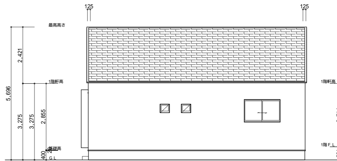
東側 立面図 S:1/100
