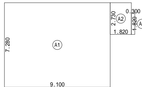
1階 床面積求積図 S:1/200
