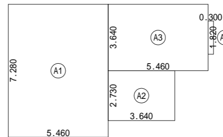
2階 床面積求積図 S:1/200
