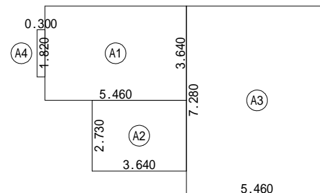
2階 床面積求積図 S:1/200
