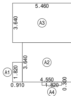
1階 床面積求積図 S:1/200
