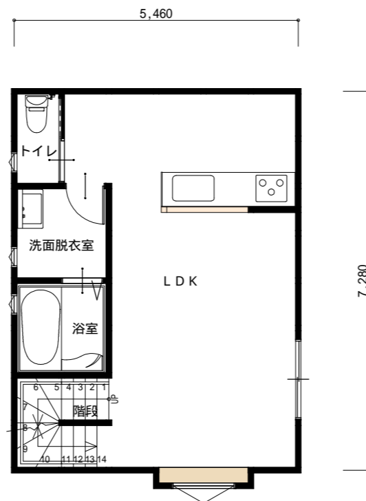
2階 平面図 S:1/100
