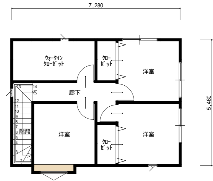
3階 平面図 S:1/100
