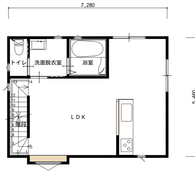
2階 平面図 S:1/100
