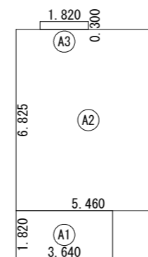
2階 床面積求積図 S:1/200
