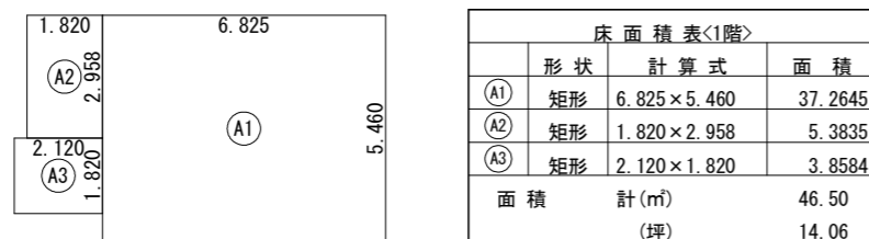
1階 床面積求積図 S:1/200
