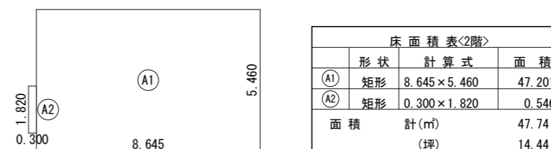
2階 床面積求積図 S:1/200
