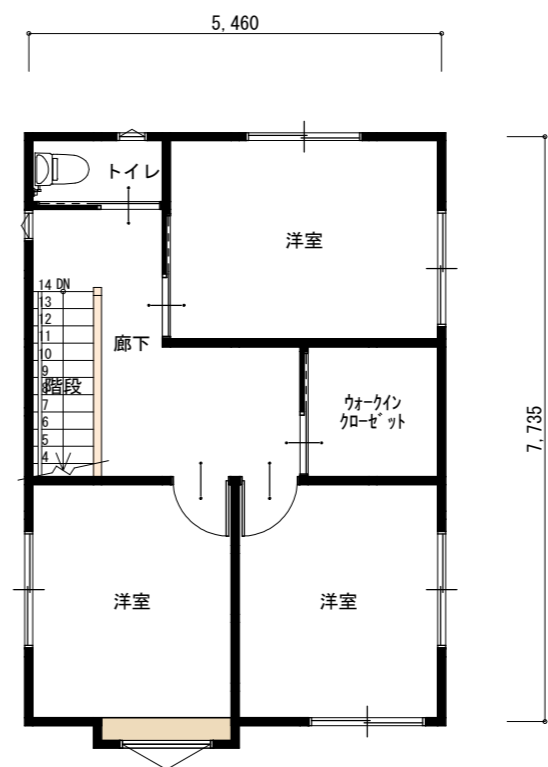
2階 平面図 S:1/100
