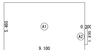
2階 床面積求積図 S:1/200
