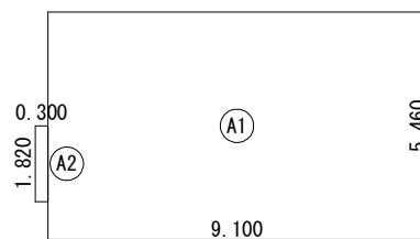
2階 床面積求積図 S:1/200
