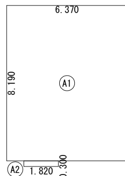
2階 床面積求積図 S:1/200
