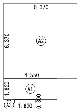
1階 床面積求積図 S:1/200
