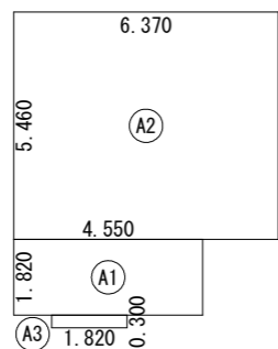
1階 床面積求積図 S:1/200
