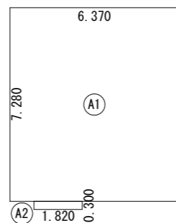
2階 床面積求積図 S:1/200
