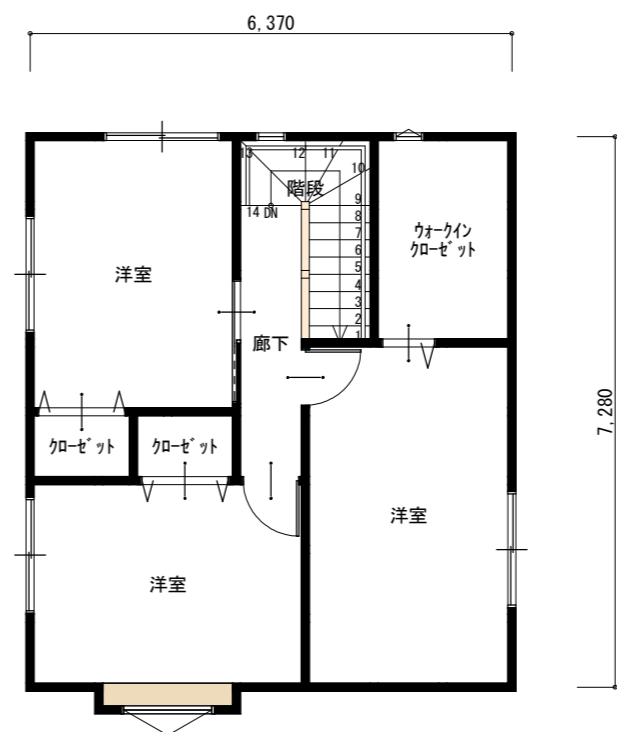
2階 平面図 S:1/100
