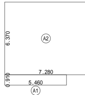
1階 床面積求積図 S:1/200
