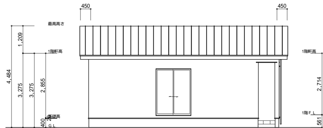
西側 立面図 S:1/100
