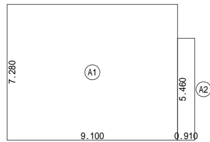
1階 床面積求積図 S:1/200
