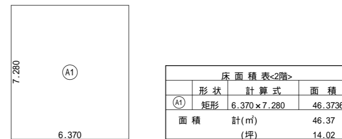
2階 平面図 S:1/100
