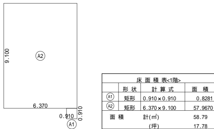
1階 床面積求積図 S:1/200
