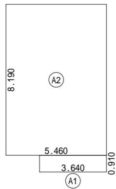
1階 床面積求積図 S:1/200
