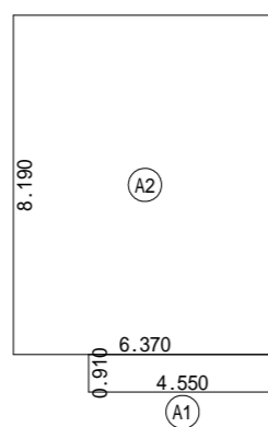
1階 床面積求積図 S:1/200
