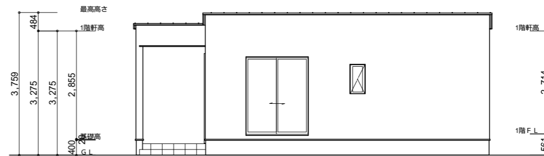
西側 立面図 S:1/100
