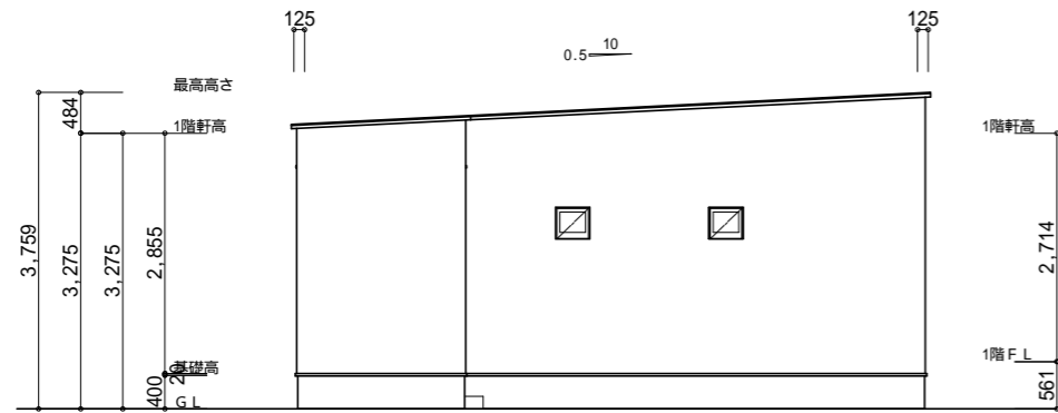
北側 立面図 S:1/100
