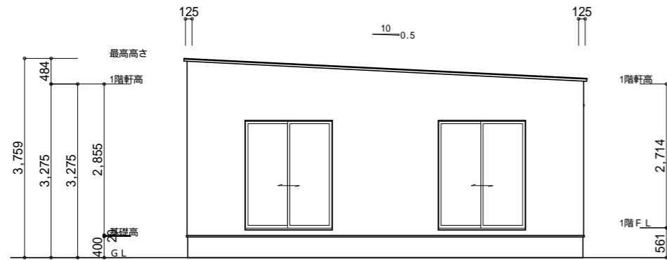
南側 立面図 S:1/100
