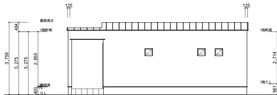
北側 立面図 S:1/100
