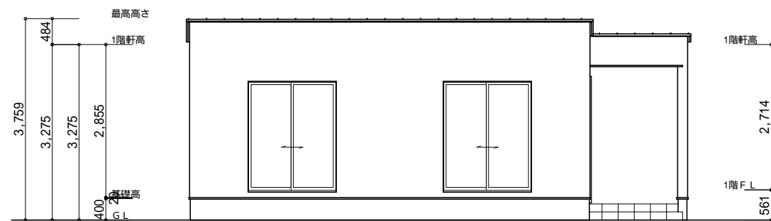
南側 立面図 S:1/100
