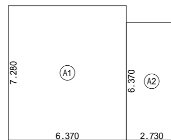
2階 床面積求積図 S:1/200
