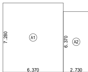
1階 床面積求積図 S:1/200
