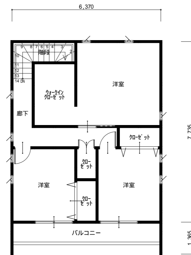
2階 平面図 S:1/100
