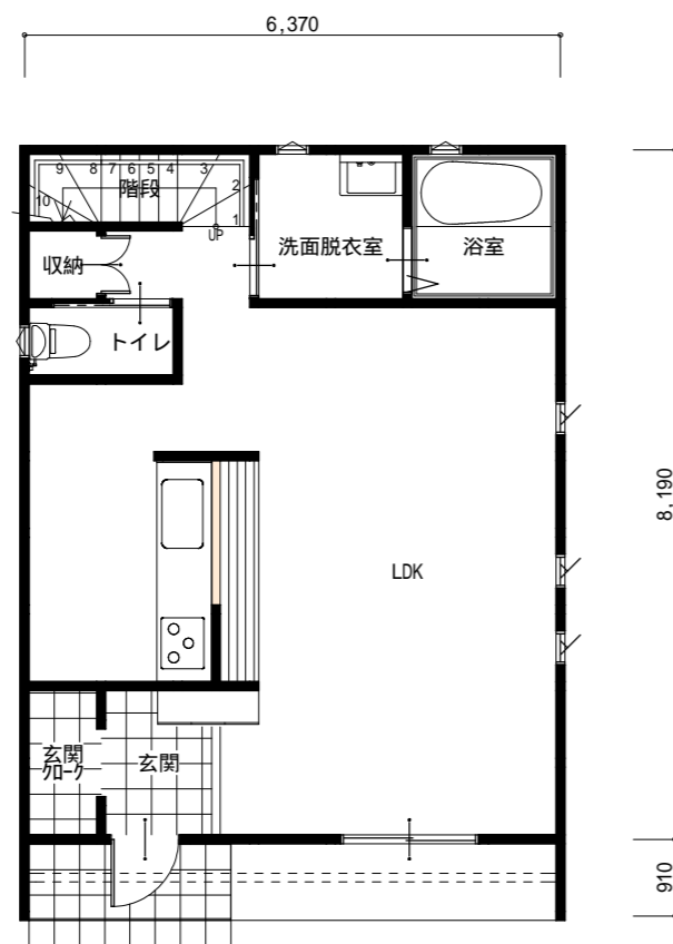
1階 平面図 S:1/100
