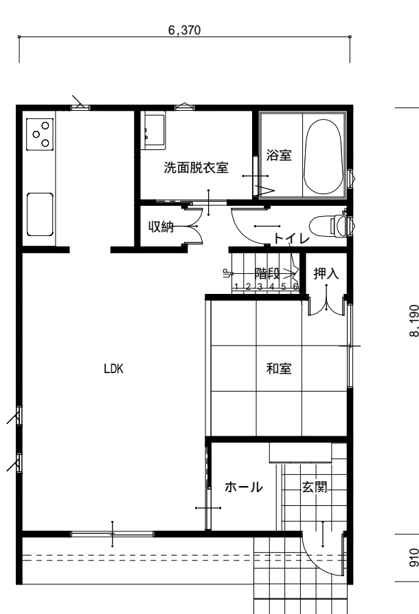
1階 平面図 S:1/100
